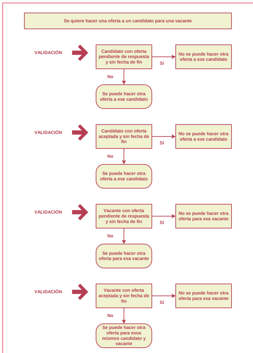
Figura 3. Validaciones sobre ofertas y vacantes
