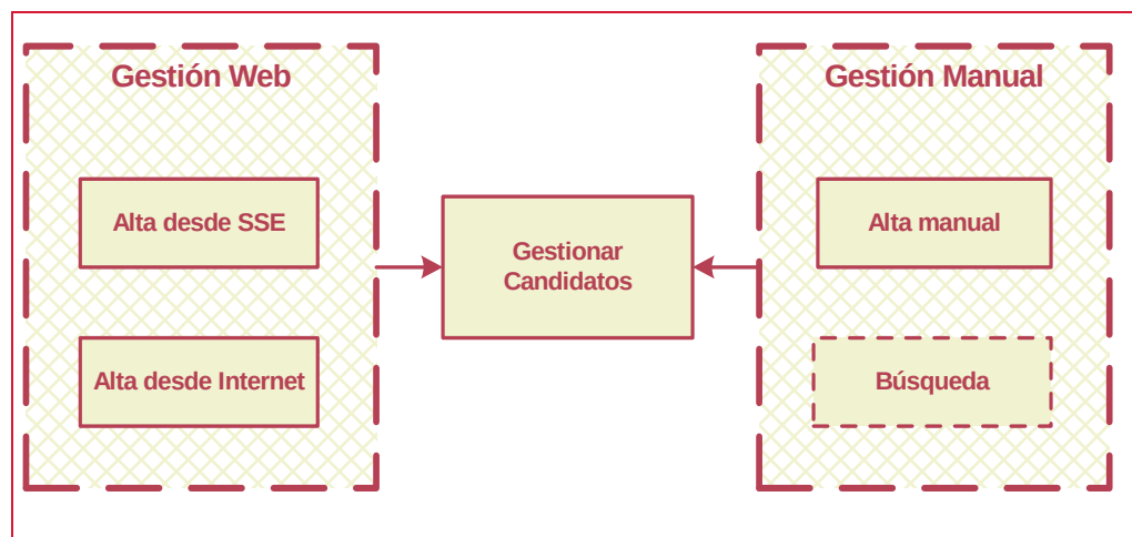
Figura 1. Funcionalidad asociada al alta de candidatos y asignación a procesos de selección
